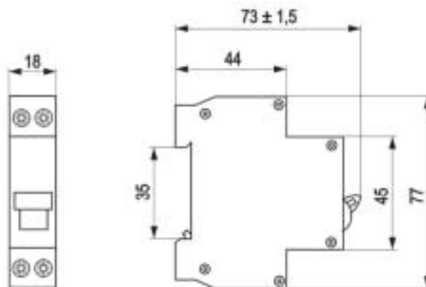
Габаритные размеры
