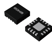
VQFN016V3030 3.00mm×3.00mm h: 1.00mm
