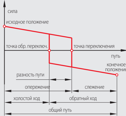
Диаграмма управления выключателя мгновенного действия
