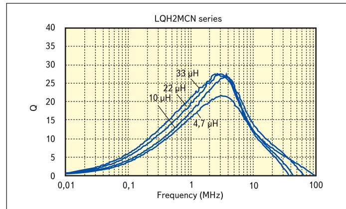
Рис. 3. Зависимость добротности Q частоты для LQH2MCN
