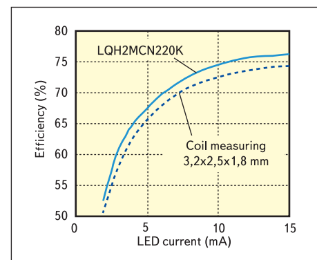
Рис. 5. Зависимость КПД от тока для тестовой схемы с использованием LQH2MCN
