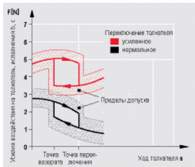
Диаграмма передачи усилия при нажатии толкателя, исполнение S800b, S800c
