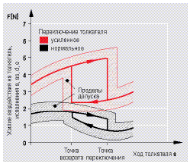
Диаграмма передачи усилия при нажатии на роликовый рычаг, исполнение S800a, S800as, S800d, S800e
