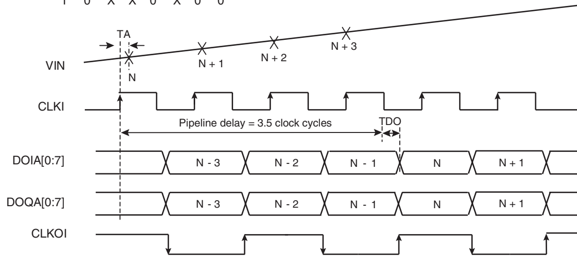
Figure 7-5. 1:1 DMUX Mode, Clock I = ADC I, Clock I = ADC Q Address: D7 D6 D5 D4 D3 D2 D1 D0 1 0 X X 0 X 0 0
